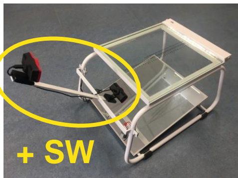
PodoCam - 2 kamery, držák, software
